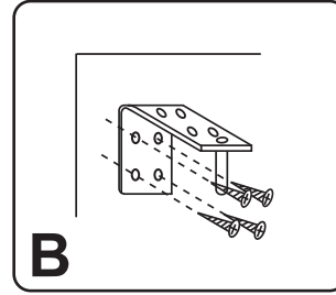
B. Montage extérieur à l'avant ou à l'extérieur du cadre de la fenêtre.
