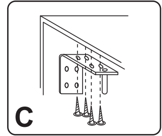
C. Montage sur une surface telle que sur la partie supérieure à l'intérieur du cadre de la fenêtre ou le plafond.
